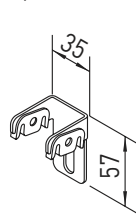
Spacer
